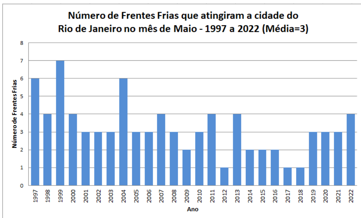
Figura 2 – Frequência anual de Sistemas Frontais que atingiram a cidade do Rio de Janeiro no mês de maio, no período entre 1997 e 2022.
