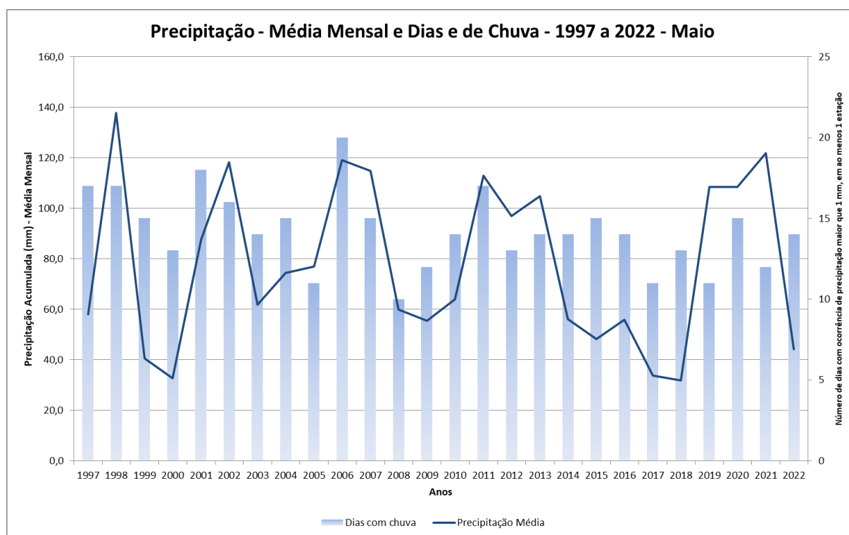
Figura 1: Precipitação média mensal (curva em azul escuro) e número de dias de chuva (barras em azul claro) para os meses de maio do período de 1997 a 2022.
