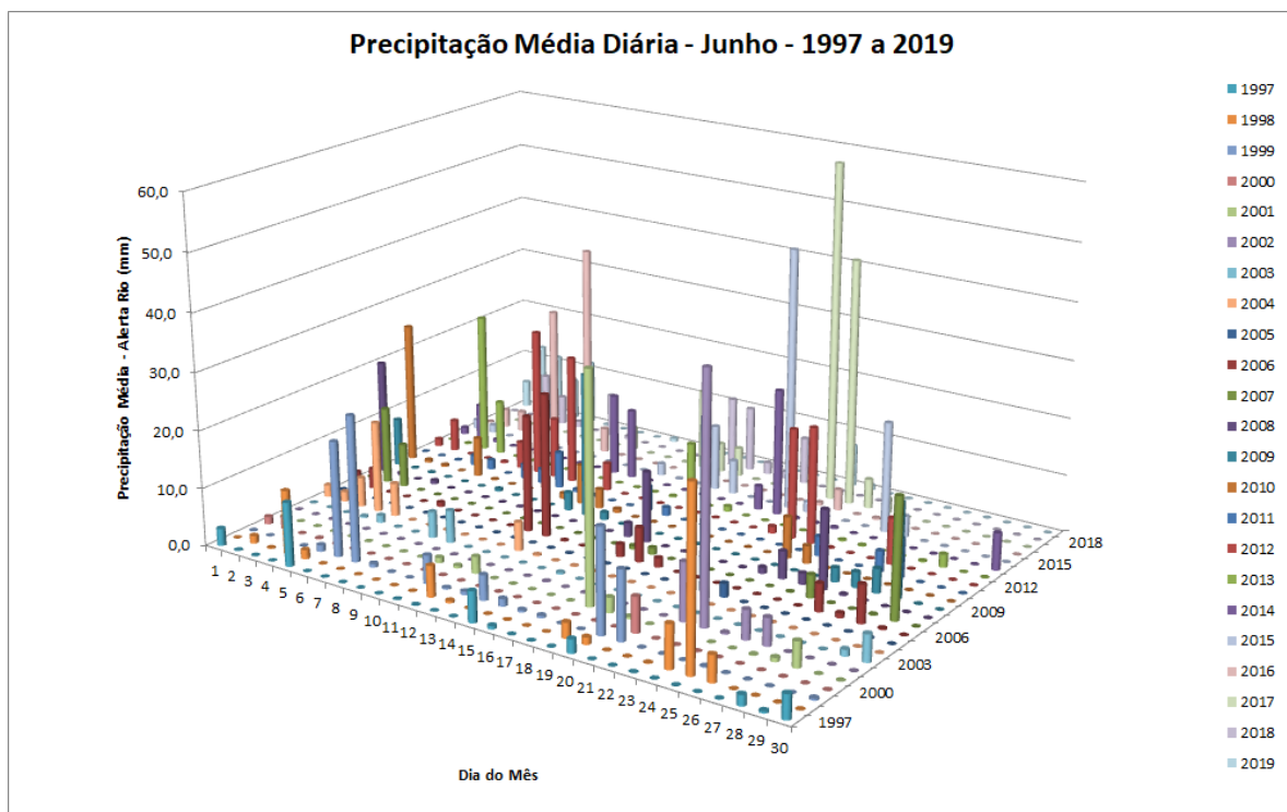
Figura 2: Precipitação média diária nas estações do Alerta Rio para cada dia do mês de junho entre os anos de 1997 e 2019.
