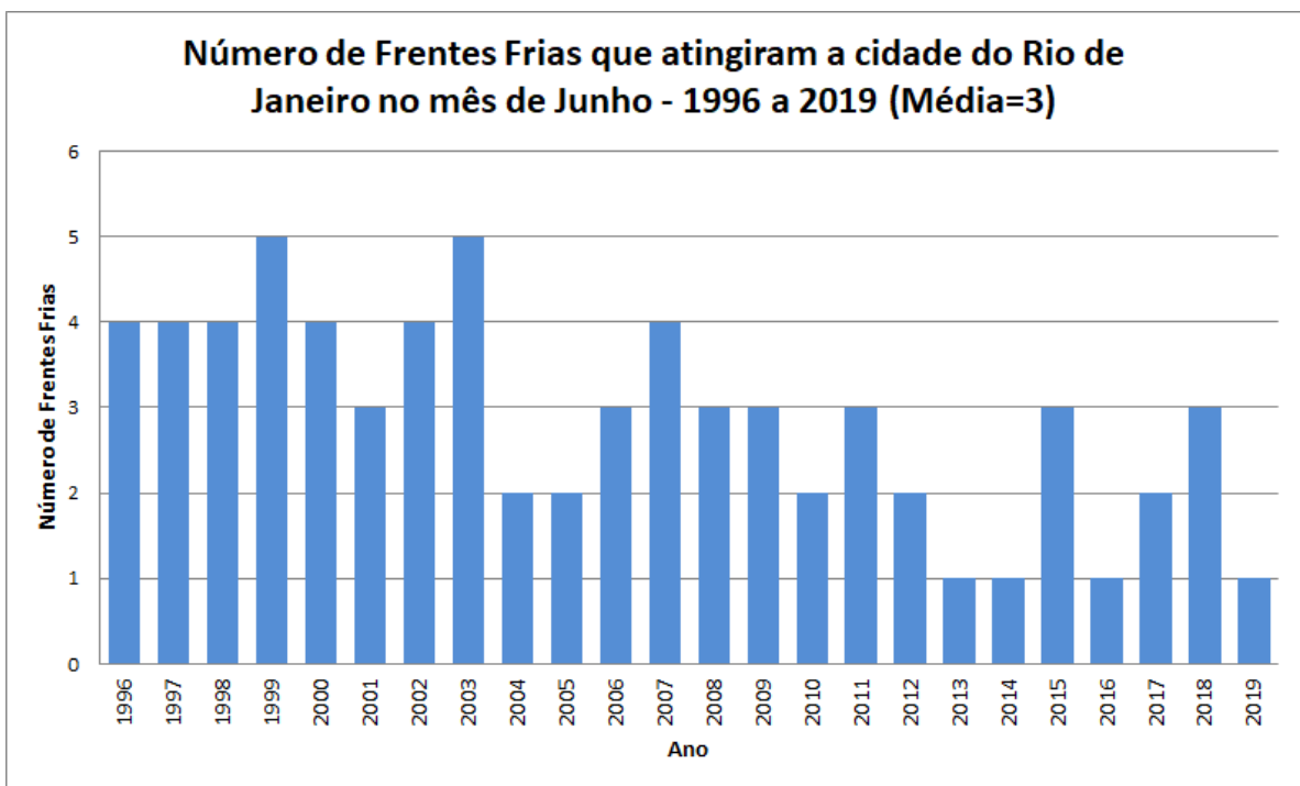
Figura 5 – Frequência anual de Sistemas Frontais que atingiram a cidade do Rio de Janeiro no mês de junho, no período entre 1996 e 2019.
