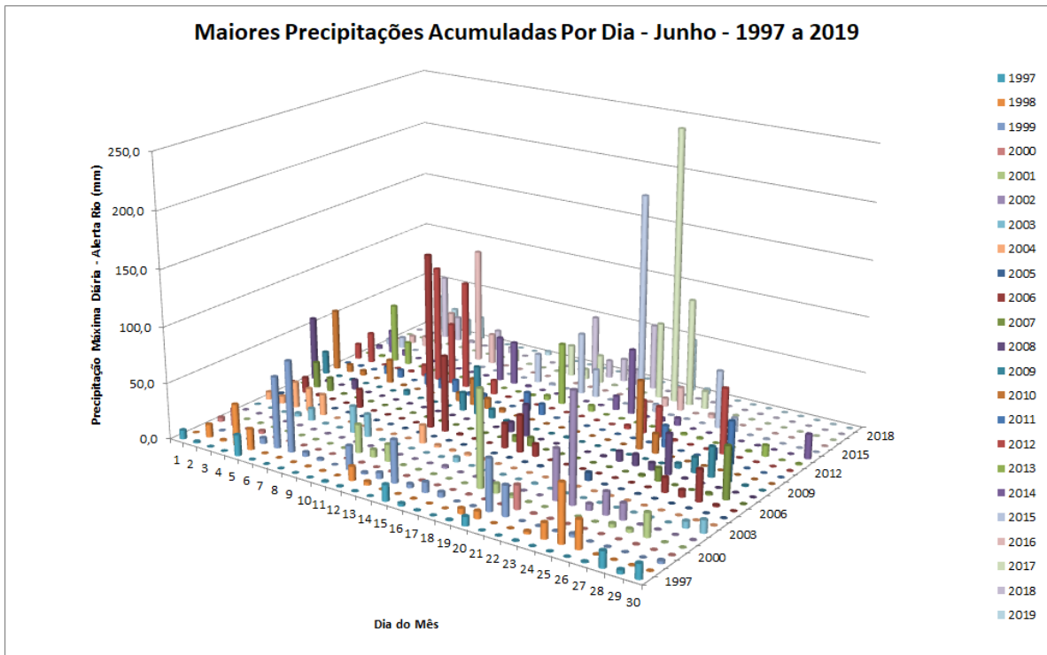
Figura 3: Maiores precipitações acumuladas por dia na rede de estações do Alerta Rio para cada dia do mês de junho entre os anos de 1997 e 2019.
