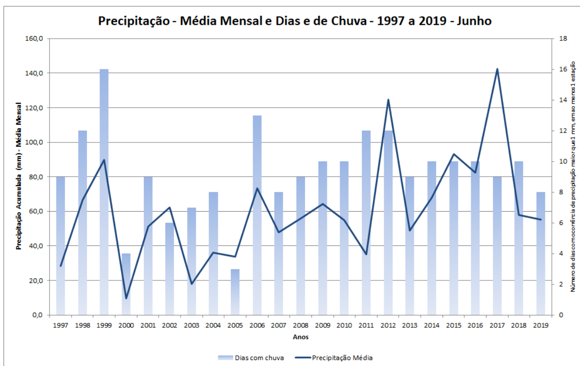
Figura 1: Precipitação média mensal (curva em azul escuro) e número de dias de chuva (barras em azul claro) para os meses de junho do período de 1997 a 2019.
