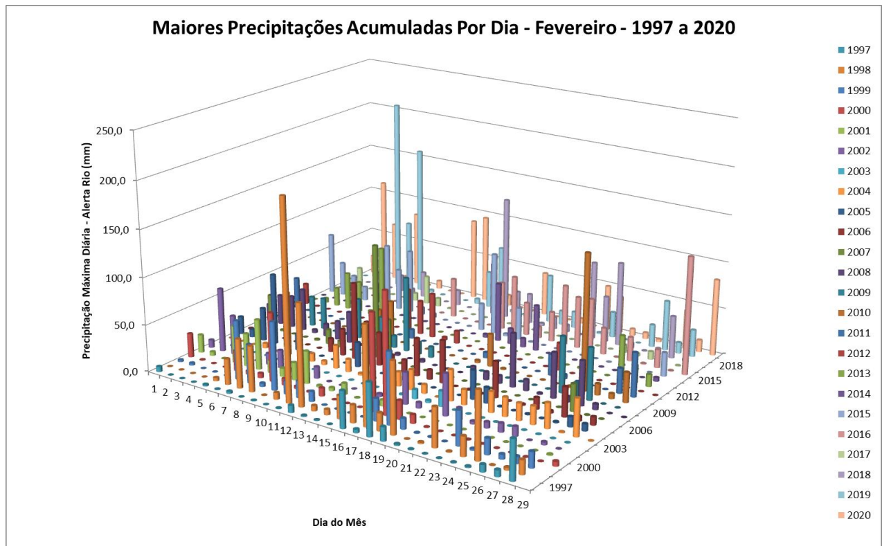
Figura 3: Maiores precipitações acumuladas por dia na rede de estações do Alerta Rio para cada dia do mês de fevereiro entre os anos de 1997 e 2020.
