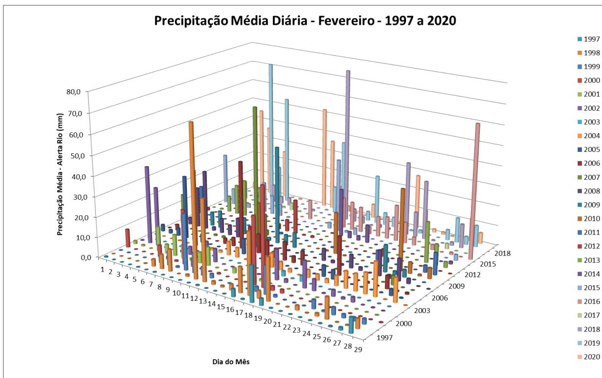
Figura 2: Precipitação média diária nas estações do Alerta Rio para cada dia do mês de fevereiro entre os anos de 1997 e 2020.
