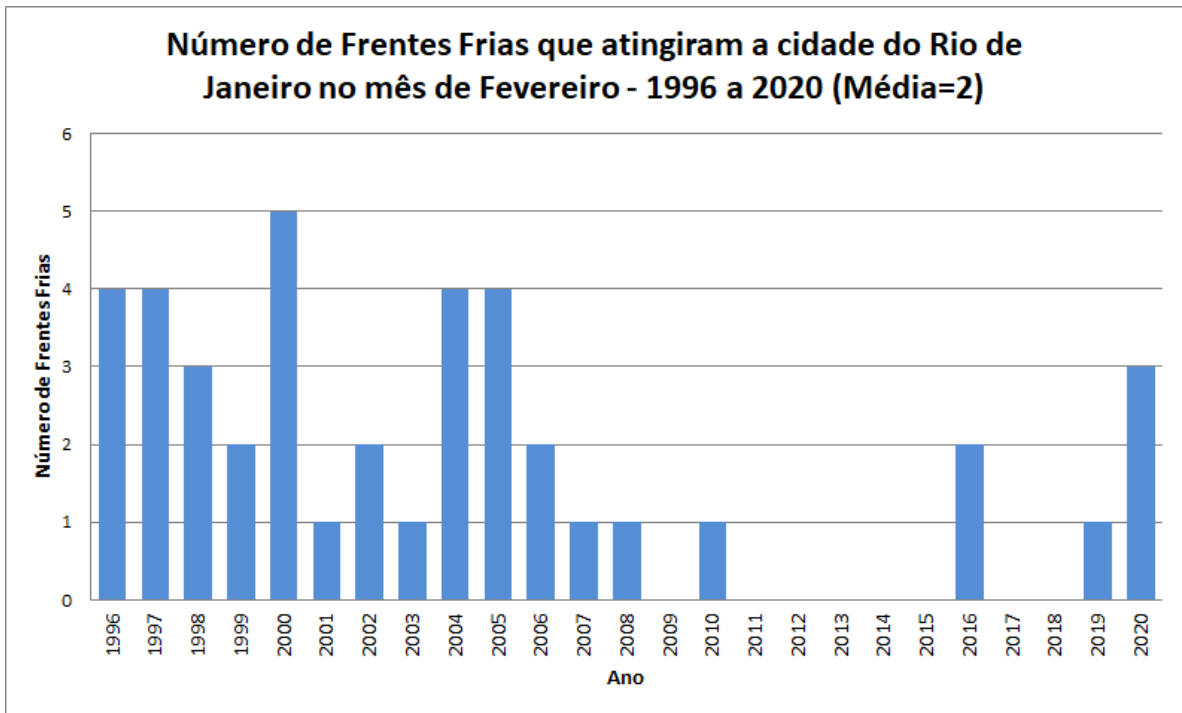
Figura 4 – Frequência anual de Sistemas Frontais que atingiram a cidade do Rio de Janeiro no mês de Fevereiro, no período entre 1996 e 2020.
