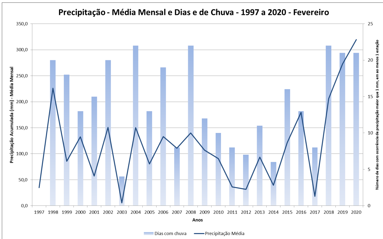
Figura 1: Precipitação média mensal (curva em azul escuro) e número de dias de chuva (barras em azul claro) para os meses de fevereiro do período de 1997 a 2020.
