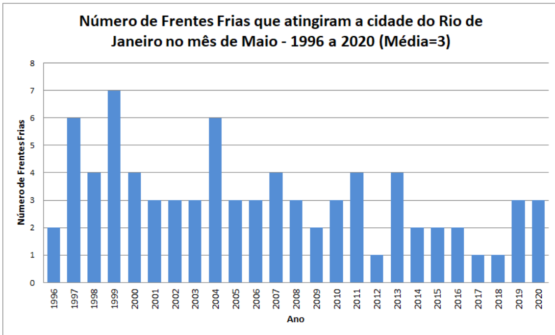
Figura 4 – Frequência anual de Sistemas Frontais que atingiram a cidade do Rio de Janeiro no mês de maio, no período entre 1996 e 2020.
