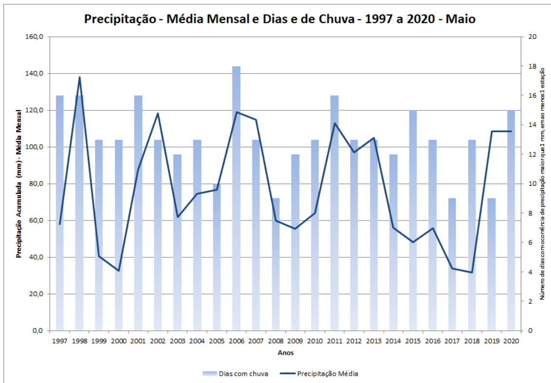
Figura 1: Precipitação média mensal (curva em azul escuro) e número de dias de chuva (barras em azul claro) para os meses de maio do período de 1997 a 2020.
