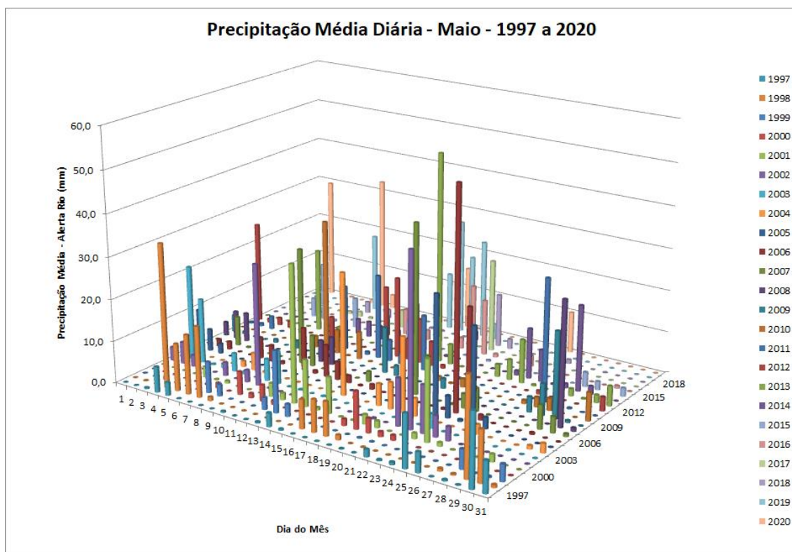
Figura 2: Precipitação média diária nas estações do Alerta Rio para cada dia do mês de maio entre os anos de 1997 e 2020.
