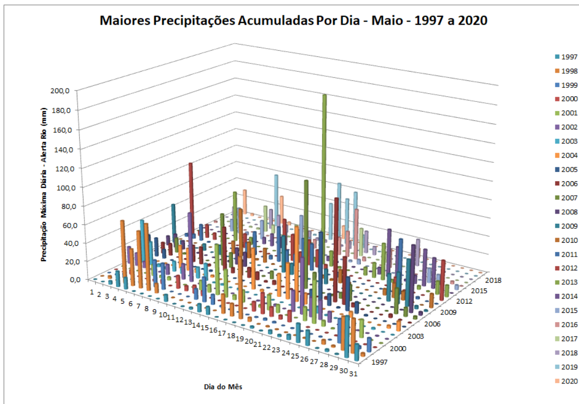
Figura 3: Maiores precipitações acumuladas por dia na rede de estações do Alerta Rio para cada dia do mês de maio entre os anos de 1997 e 2020.
