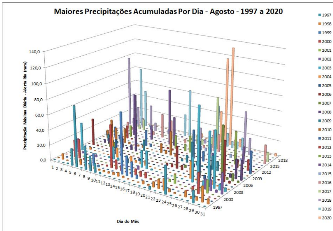
Figura 3: Maidores precipitações acumuladas por dia na rede de estações do Alerta Rio para cada dia do mês de agosto entre os anos de 1997 e 2020.
