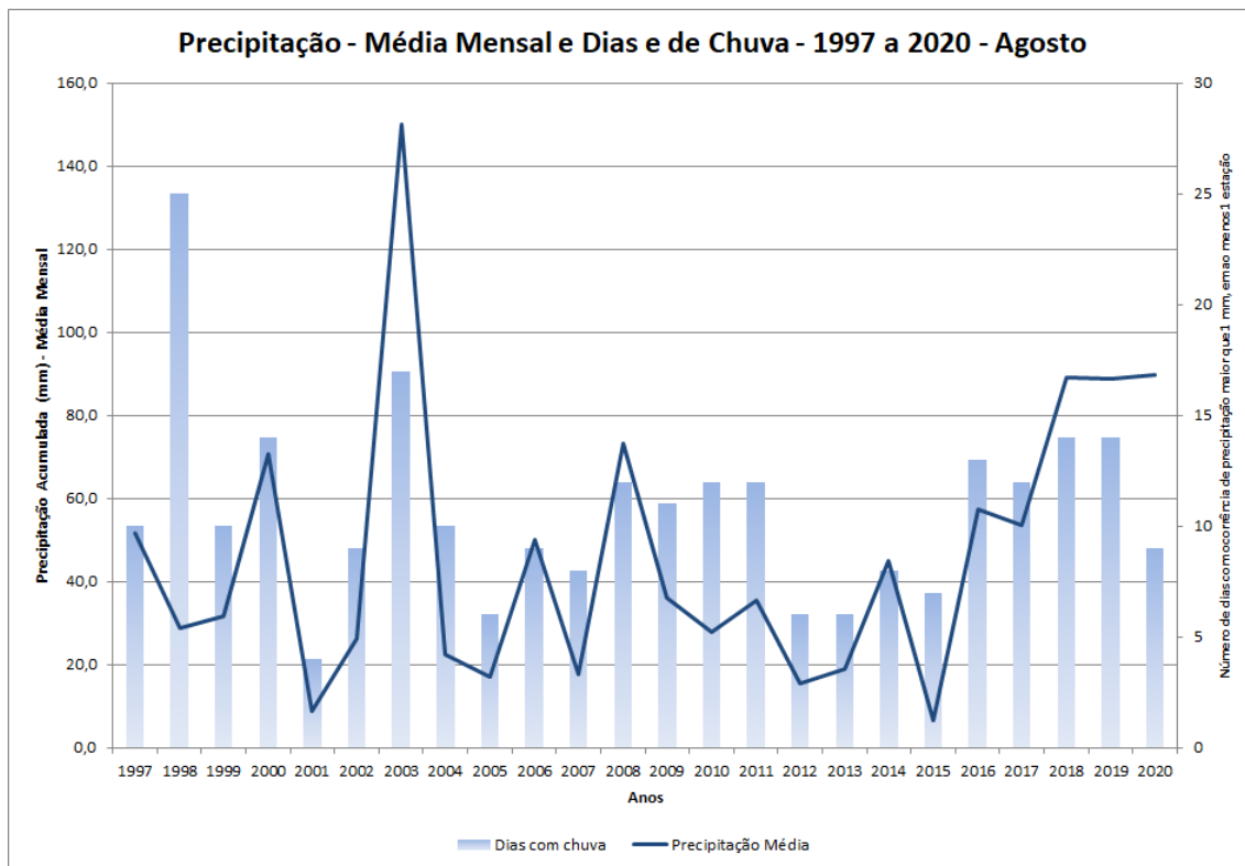
Figura 1: Precipitação média mensal (curva em azul escuro) e número de dias de chuva (barras em azul claro) para os meses de agosto do período de 1997 a 2020.
