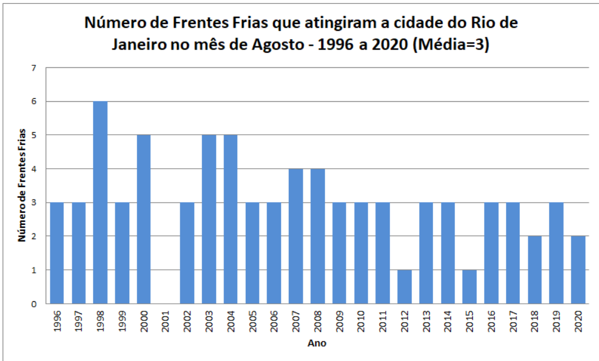
Figura 4 – Frequência anual de Sistemas Frontais que atingiram a cidade do Rio de Janeiro no mês de agosto, no período entre 1996 e 2020.
