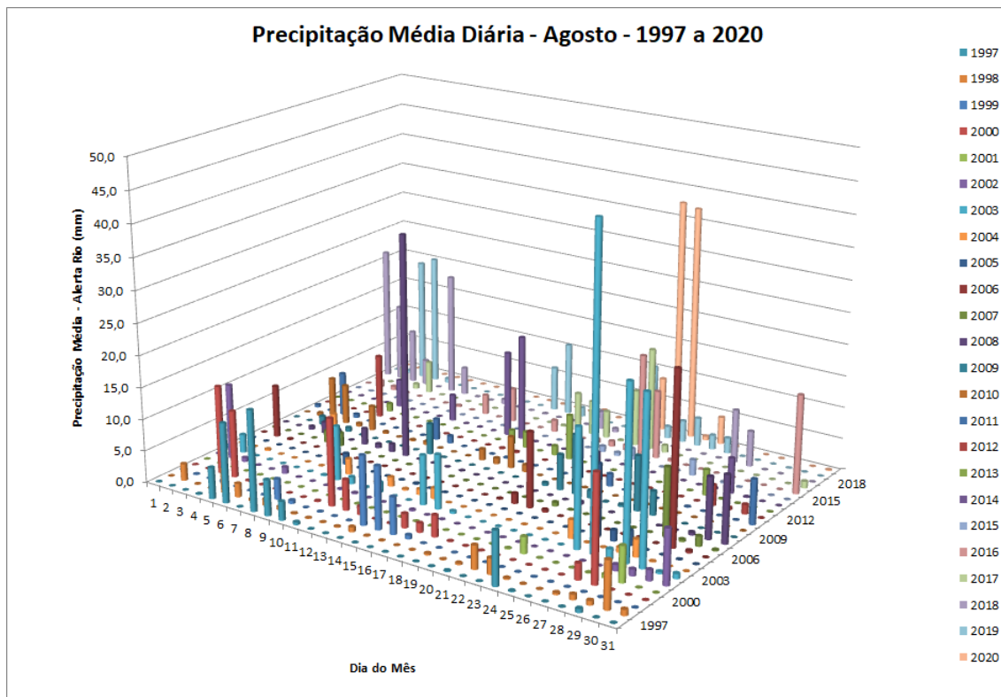
Figura 2: Precipitação média diária nas estações do Alerta Rio para cada dia do mês de agosto entre os anos de 1997 e 2020.
