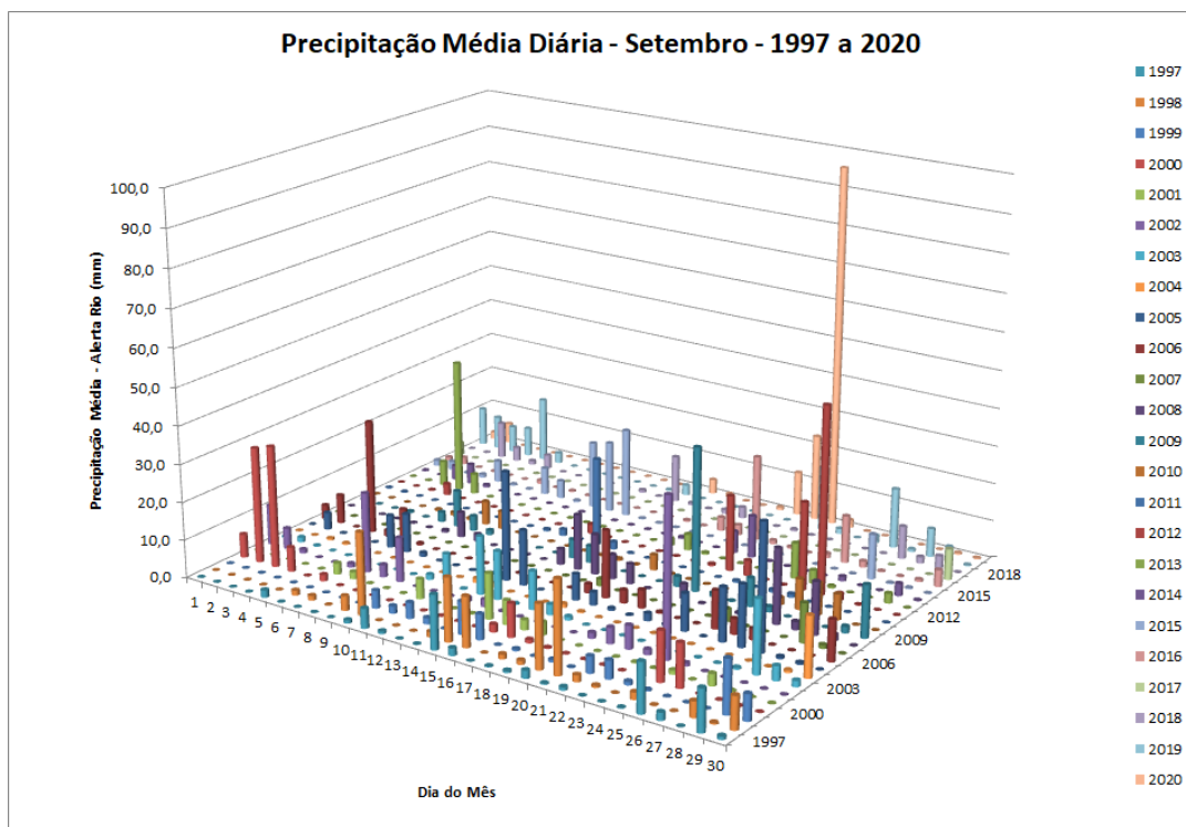
Figura 2: Precipitação média diária nas estações do Alerta Rio para cada dia do mês de setembro entre os anos de 1997 e 2020.
