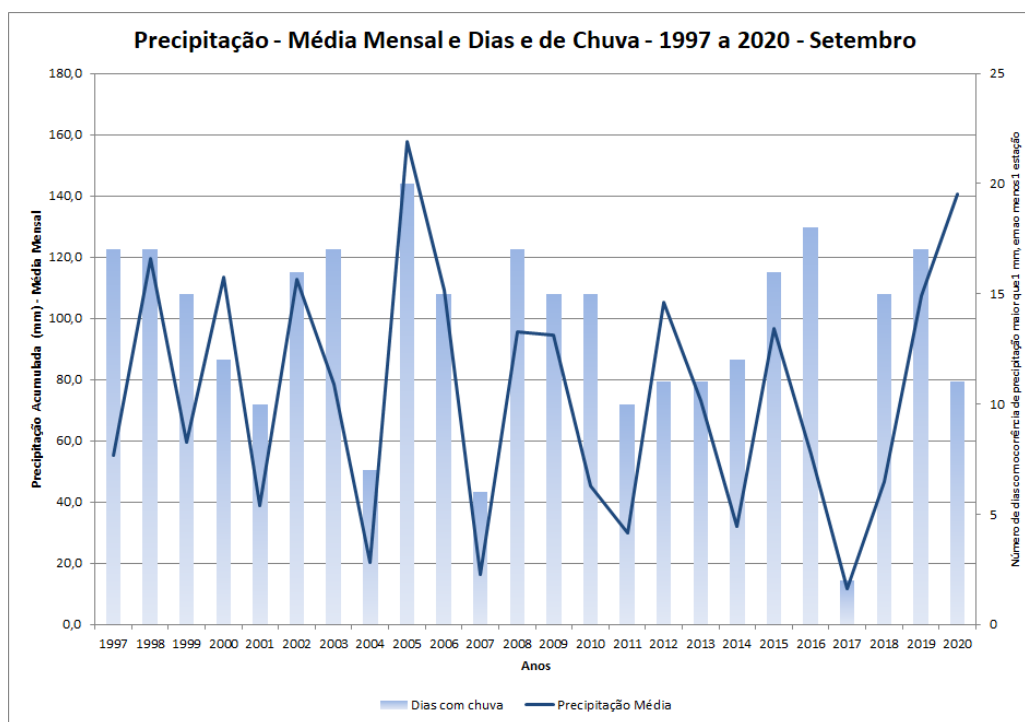
Figura 1: Precipitação média mensal (curva em azul escuro) e número de dias de chuva (barras em azul claro) para os meses de setembro do período de 1997 a 2020.
