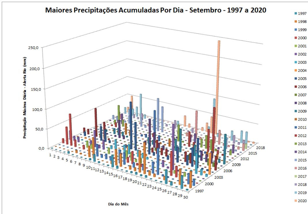
Figura 3: Maiores precipitações acumuladas por dia na rede de estações do Alerta Rio para cada dia do mês de setembro entre os anos de 1997 e 2020.
