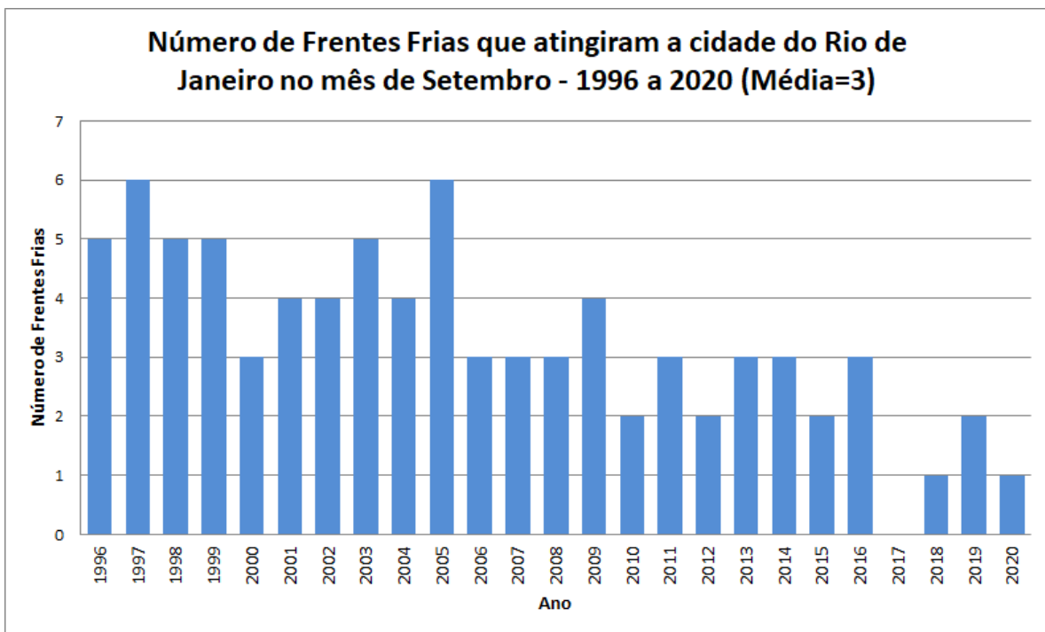
Figura 4 – Frequência anual de Sistemas Frontais que atingiram a cidade do Rio de Janeiro no mês de setembro, no período entre 1996 e 2020.
