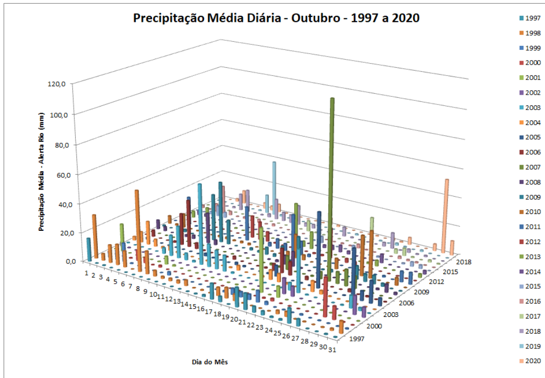
Figura 2: Precipitação média diária nas estações do Alerta Rio para cada dia do mês de outubro entre os anos de 1997 e 2020.
