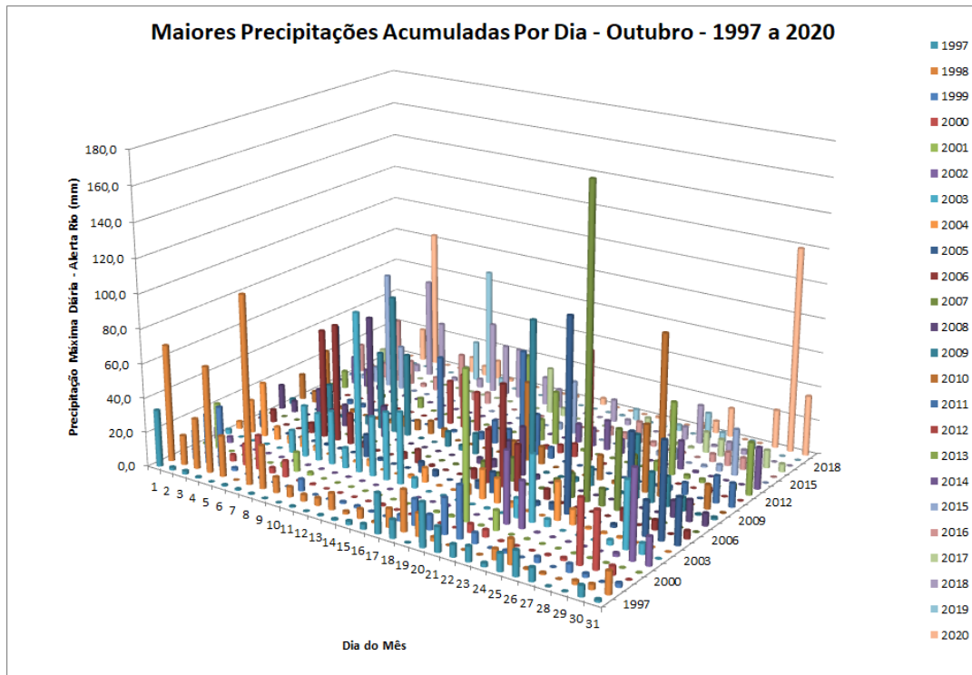
Figura 3: Maiores precipitações acumuladas por dia na rede de estações do Alerta Rio para cada dia do mês de outubro entre os anos de 1997 e 2020.
