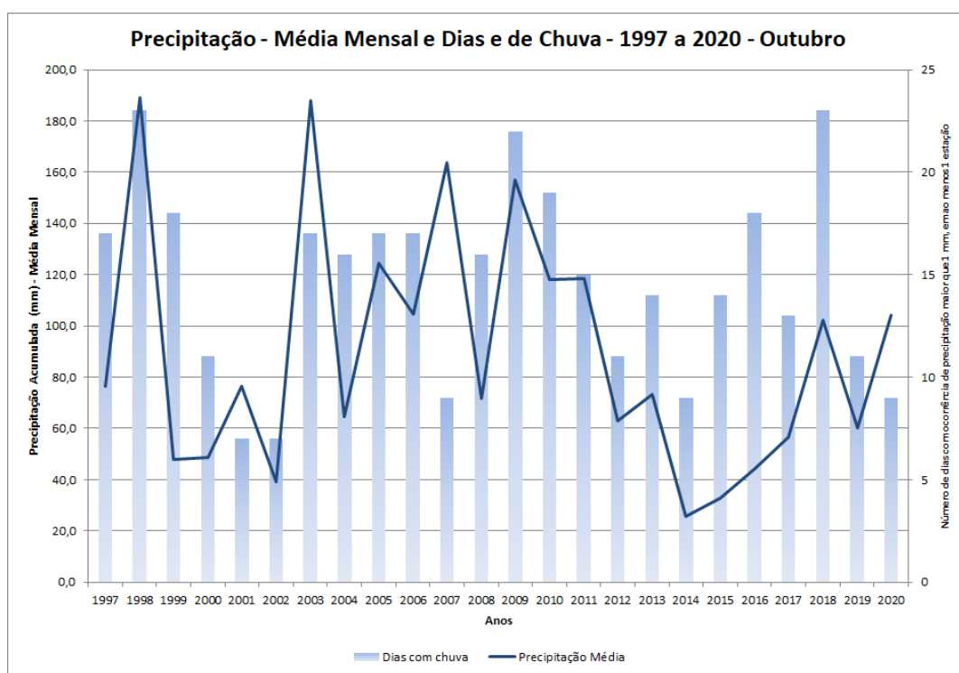
Figura 1: Precipitação média mensal (curva em azul escuro) e número de dias de chuva (barras em azul claro) para os meses de outubro do período de 1997 a 2020.
