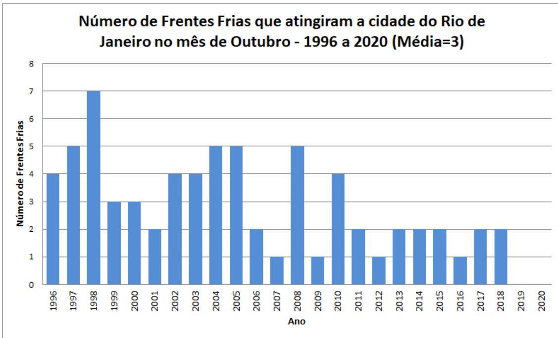
Figura 4 – Frequência anual de Sistemas Frontais que atingiram a cidade do Rio de Janeiro no mês de outubro, no período entre 1996 e 2020.
