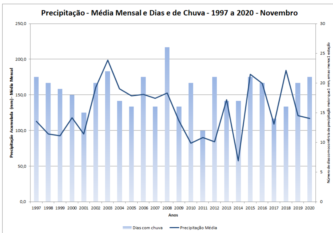
Figura 1: Precipitação média mensal (curva em azul escuro) e número de dias de chuva (barras em azul claro) para os meses de novembro do período de 1997 a 2020.
