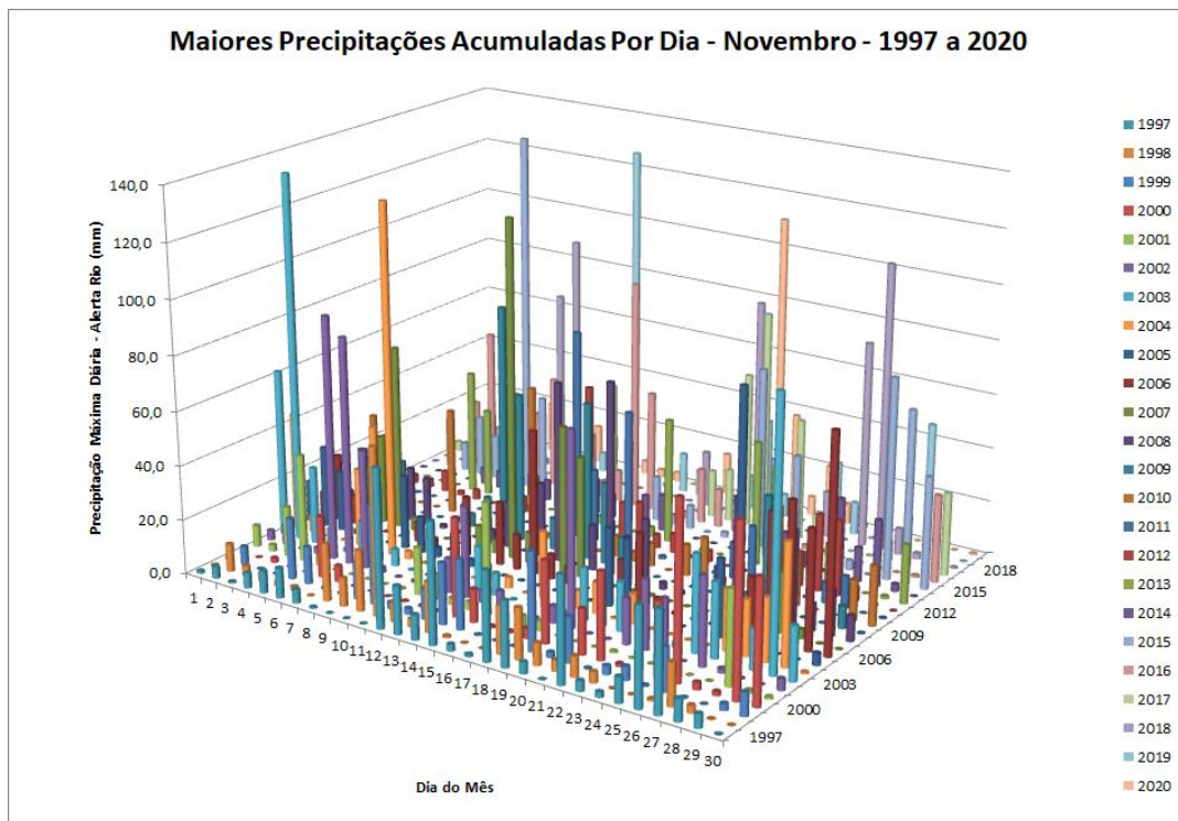
Figura 3: Maiores precipitações acumuladas por dia na rede de estações do Alerta Rio para cada dia do mês de novembro entre os anos de 1997 e 2020.
