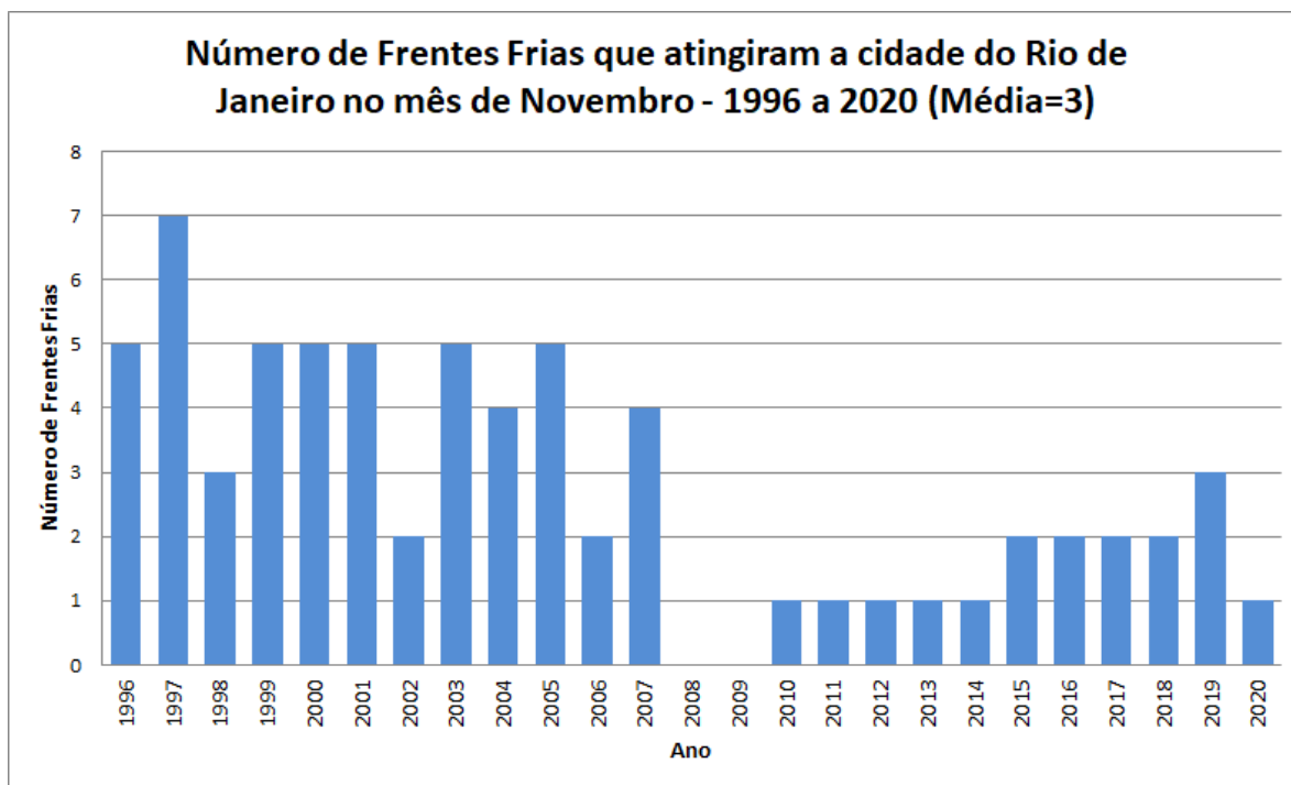
Figura 4 – Frequência anual de Sistemas Frontais que atingiram a cidade do Rio de Janeiro no mês de novembro, no período entre 1996 e 2020.
