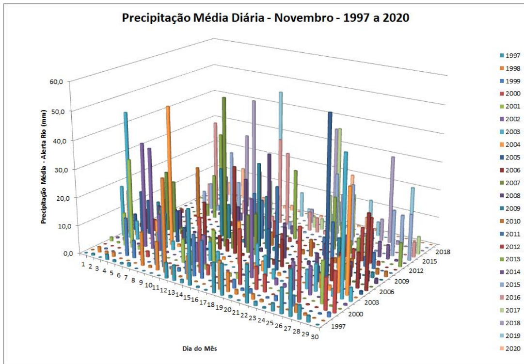
Figura 2: Precipitação média diária nas estações do Alerta Rio para cada dia do mês de novembro entre os anos de 1997 e 2020.
