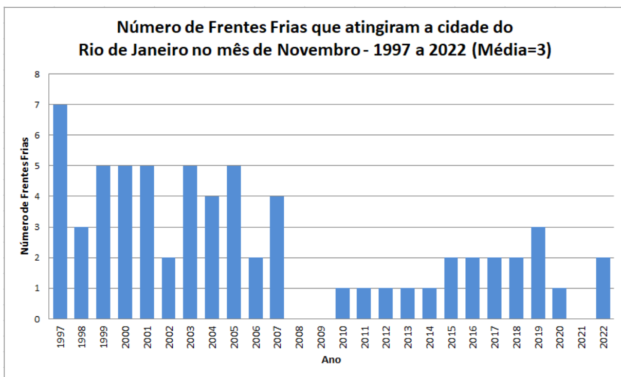
Figura 2 – Frequência anual de Sistemas Frontais que atingiram a cidade do Rio de Janeiro no mês de novembro, no período entre 1997 e 2022.
