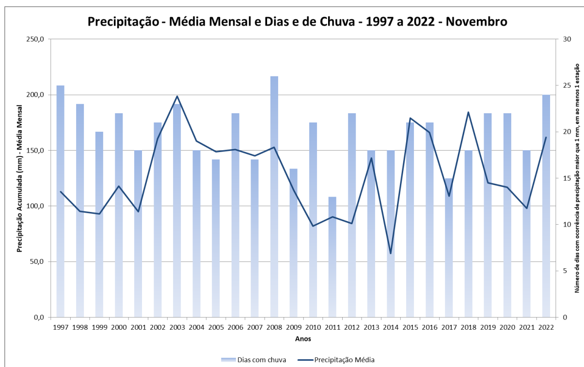
Figura 1: Precipitação média mensal (curva em azul escuro) e número de dias de chuva (barras em azul claro) para os meses de novembro do período de 1997 a 2022.
